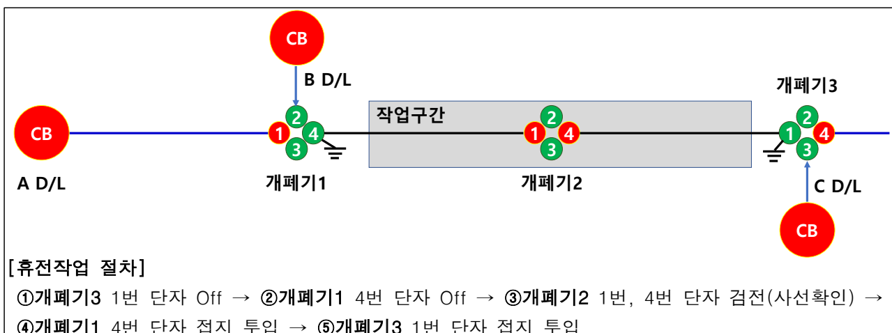
[그림 1] 배전선로 휴전작업 개념도
